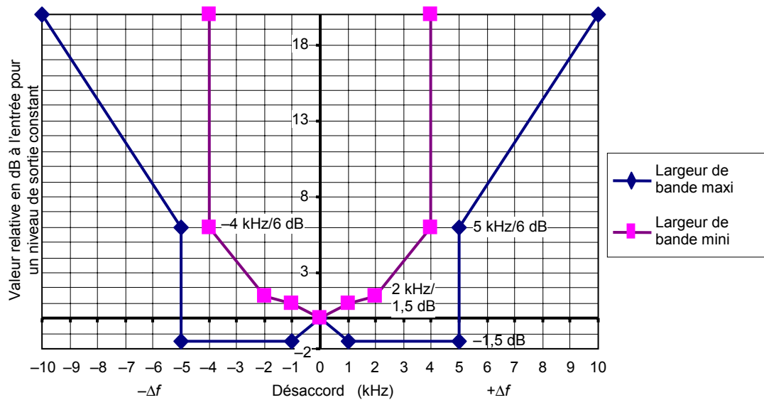
Figure 2b) – Limites de la sélectivité globale – Bande passante (voir 4.5.1, 5.6, 6.6, 7.6) (Bande B)
