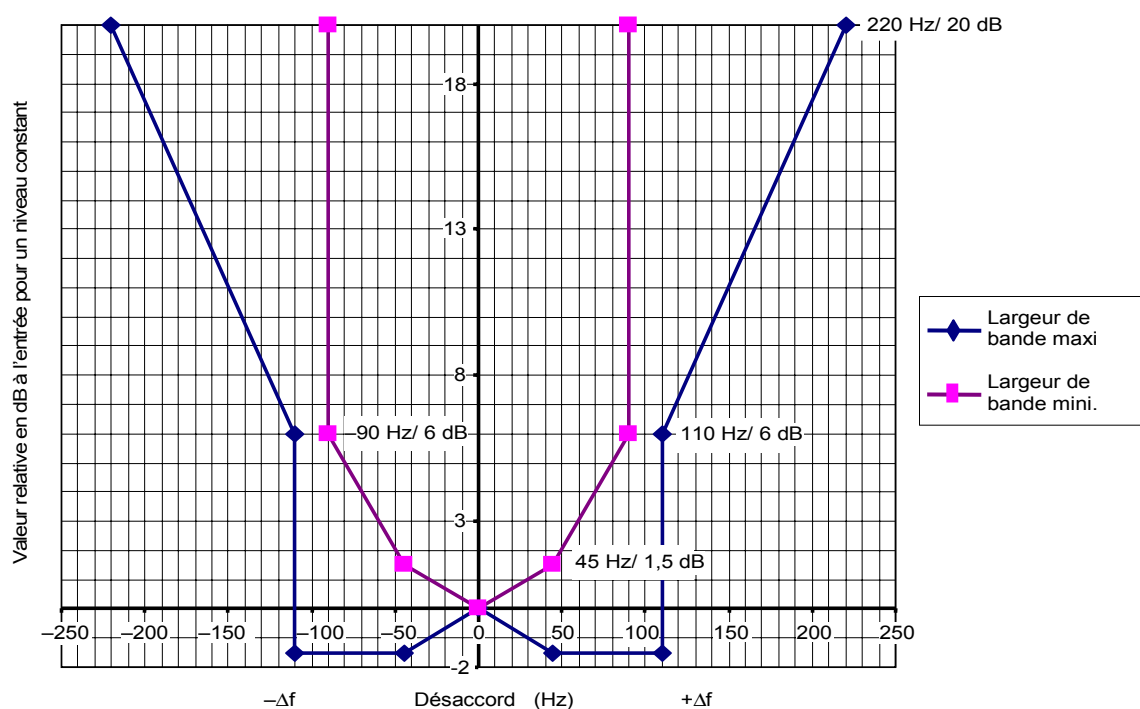
Figure 2a) – Limites de la sélectivité globale – Bande passante (voir 4.5.1, 5.6, 6.6, 7.6) (Bande A)
